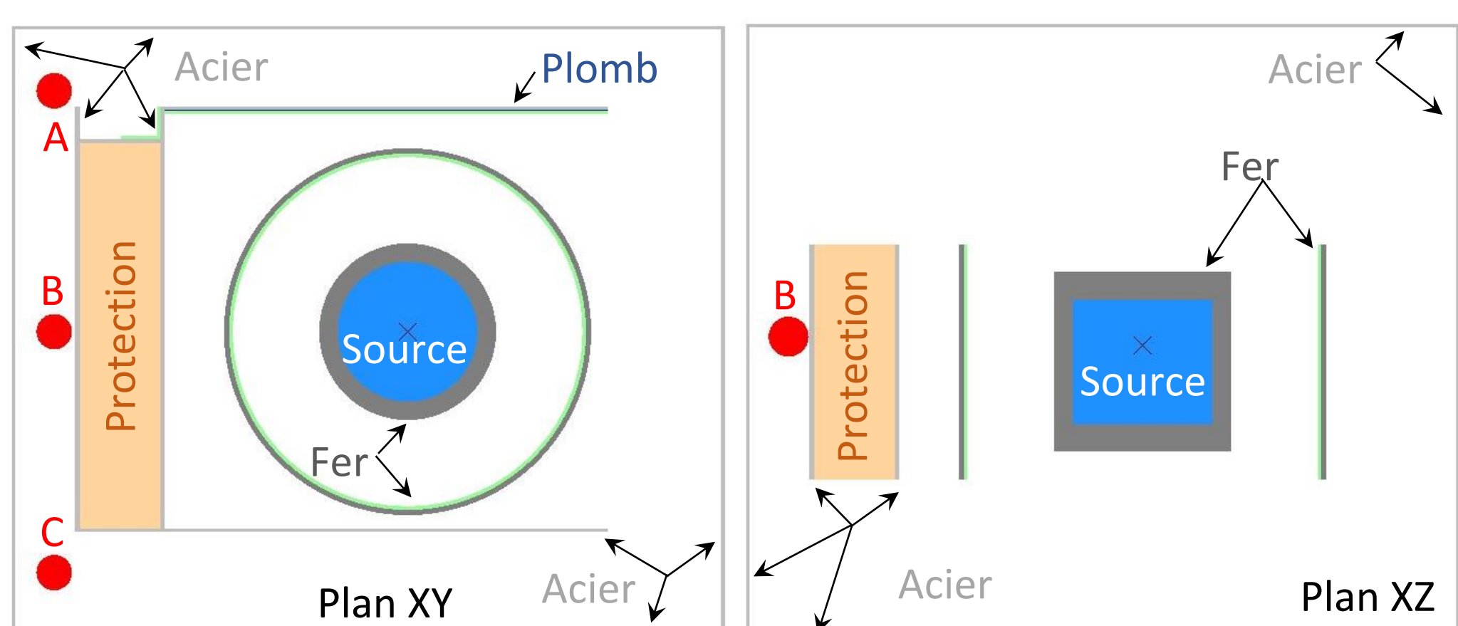
Coupes (XY) et (XZ) d'une scène de calculs de DED \gamma à proximité d'une source
