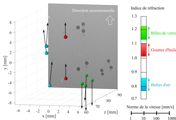
Figure 5: Reconstruction d'un hologramme de la série de résultats présentés en figure 4 - Le code couleur des particules indique la composition.
