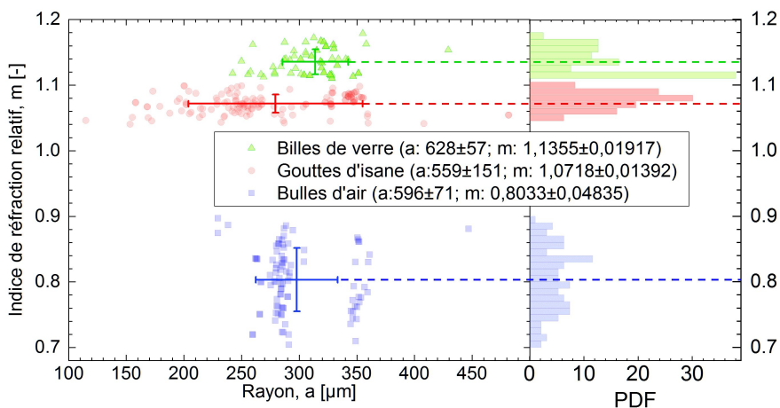
Figure 4: (a) Corrélation entre l'indice de réfraction relatif (composition) et le rayon des particules mesurés expérimentalement sur un flux de bulles d'air, de gouttes d'Isane et de billes de verre. (b) Distributions (PDF) correspondantes pour les indices de réfraction .
