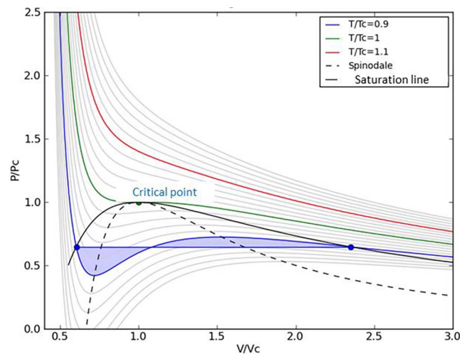
Fig. 33. Van der Waals gas.
