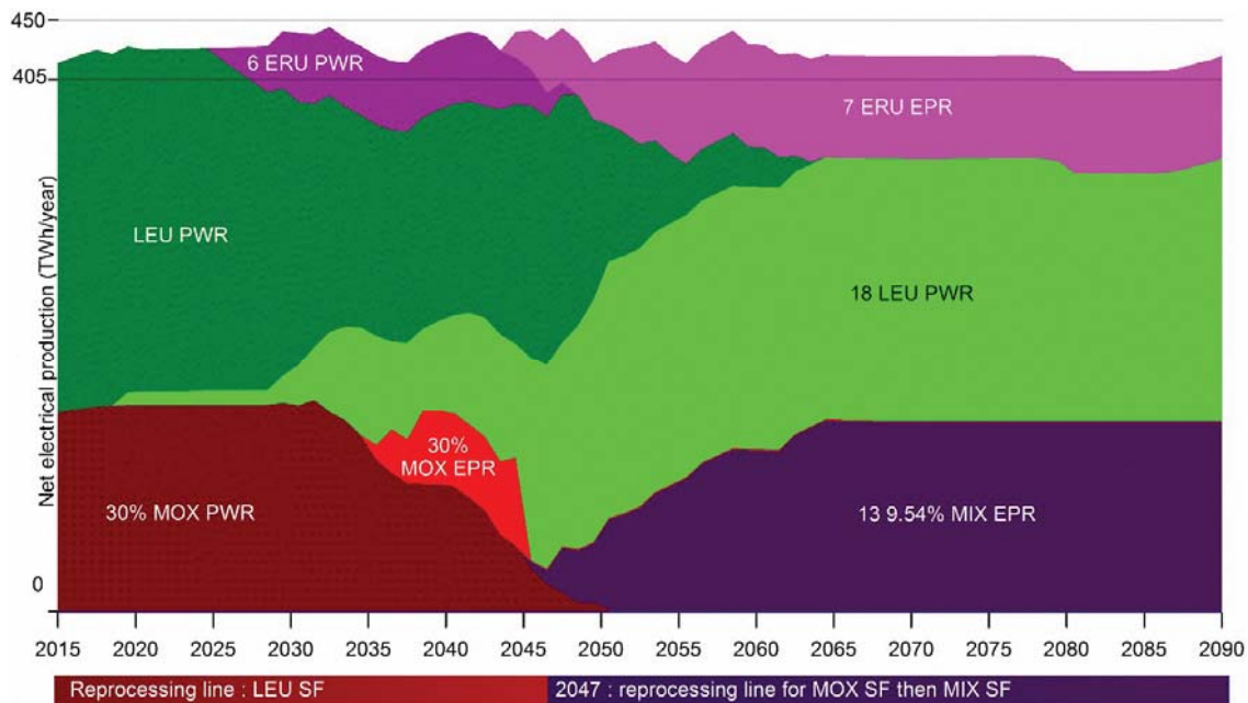
Fig. 4. Scenario 9.54% MIX with ERU.
