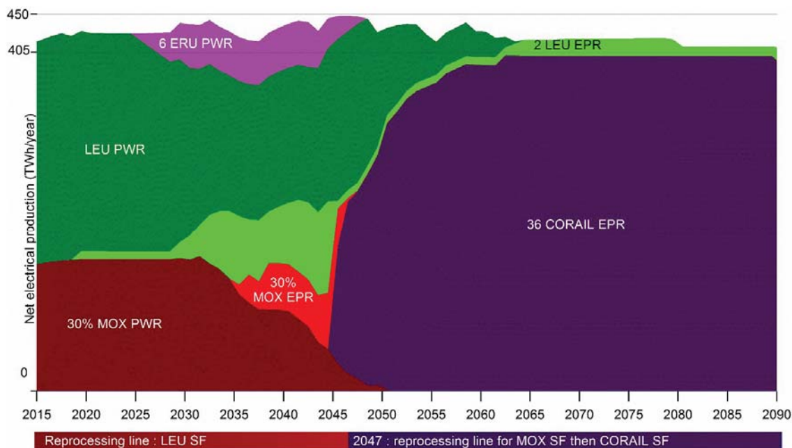
Fig. 2. Scenario CORAIL.
