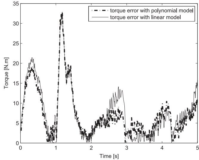
Fig. 9. High preload.
