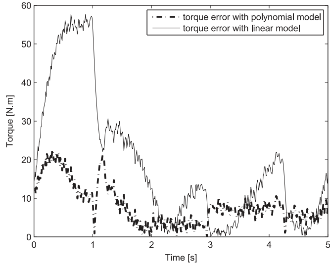
Fig. 8. Low preload.
