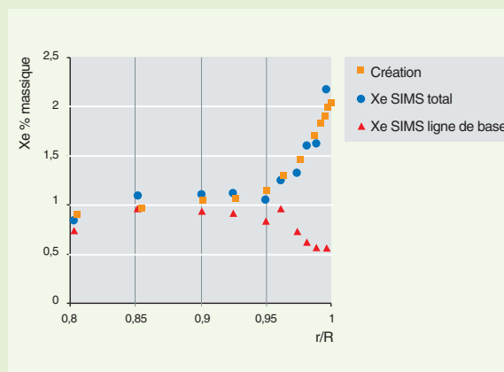
Fig. 29. Profils de concentration en xénon mesuré au SIMS en périphérie d'une pastille d' \text{UO}_2 irradiée à 60 GWj/t. L'essentiel du gaz sorti des grains (écart entre des carrés et les triangles) est retenu dans les bulles (cercles).
