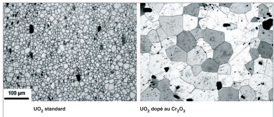
Fig. 47. Tailles des grains dans un UO 2 dopé à l'oxyde de chrome, comparée à celle dans un UO 2 standard.
