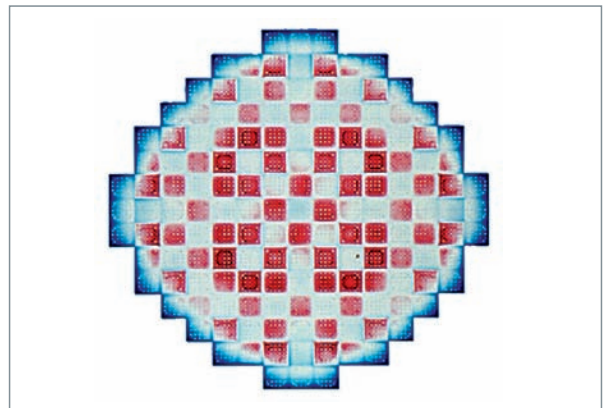
Fig. 71. Distribution de puissance calculée pour un réacteur recyclant du plutonium.
