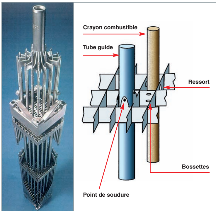
Fig. 49. Assemblage combustible + grappe de contrôle. Schéma de principe d'une cellule de grille AFA.
