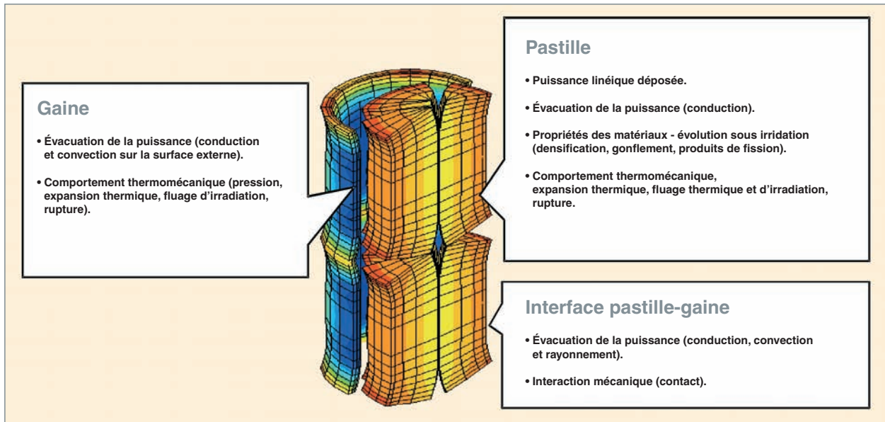
Fig. 43. Modélisation thermo-mécanique du combustible REP.
