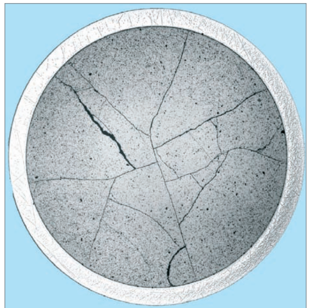
Fig. 86. Micrographie radiale d'un combustible nucléaire usé (microscopie optique) mettant en évidence l'existence de fractures radiales apparues lors de l'irradiation, sous l'effet des gradients de température.
