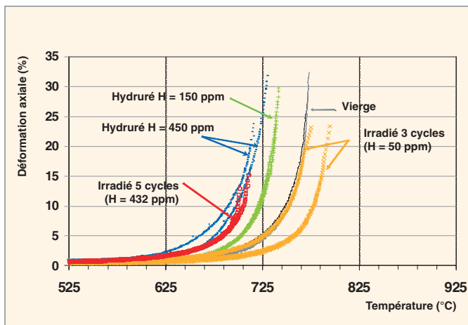
Fig. 60. Fluage du Zy-4 préhydraté et/ou irradié lors d'une rampe à 100°C/s sous chargement uni-axial de 80MPa [5].
