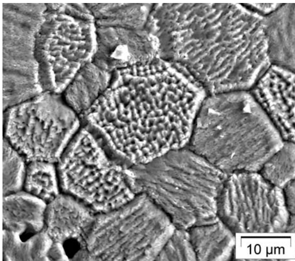
Fig. 24. Surface d'un évidement en extrémité de pastille, mise en évidence de l'évolution de la surface des grains sous irradiation et de la différence de cette évolution suivant l'orientation cristalline.
