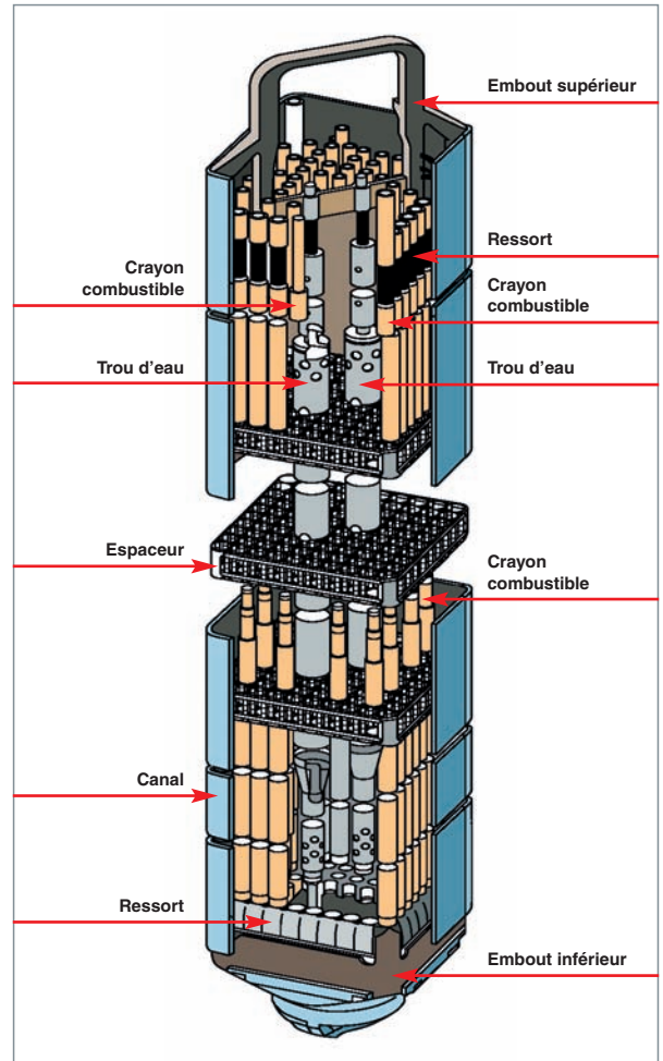
Fig. 91. Assemblage combustible pour réacteur à eau bouillante.
