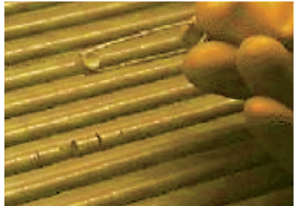
Fig. 3. Pastilles de combustible MOX, prêtes à être « engagées ».
