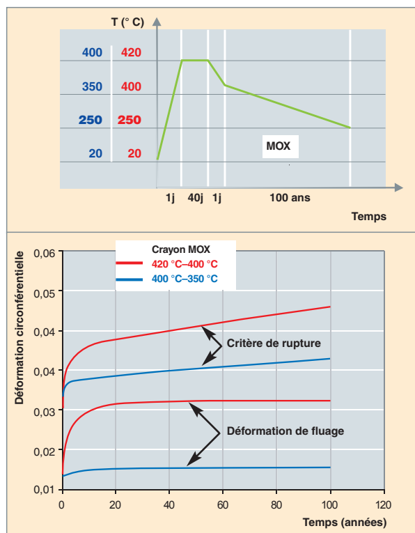
Fig. 89. Évaluation de la déformation et des marges à la rupture pour un crayon MOX en entreposage en supposant un relâchement initial de gaz de fraction très pénalisant de 18 % (mais pas de relâchement additionnel).
