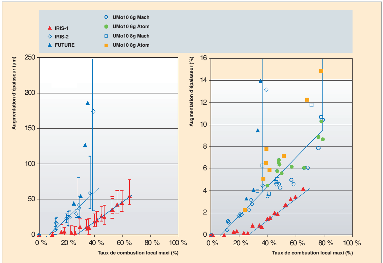
Fig. 127. Augmentation de l'épaisseur des plaques en fonction du taux de combustion a). Essais français, b). Essais intégrant les résultats de ANL.
