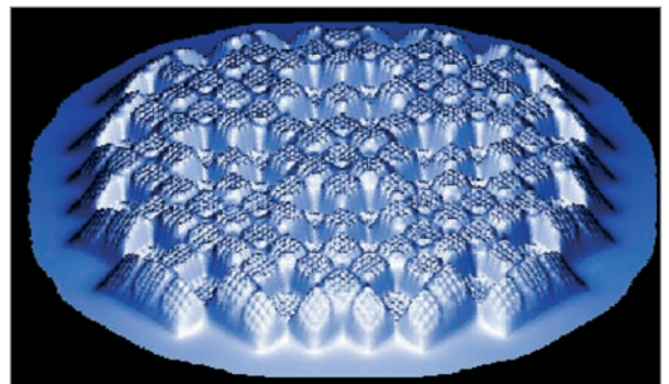
Fig. 72. Distribution du flux des neutrons thermiques dans un cœur chargé avec des assemblages MOX.
