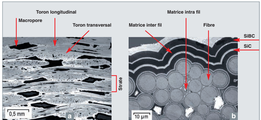
Fig. 122. Images au MEB d'un composite céramique SiC/SiC fibré (LCTS Bordeaux).
