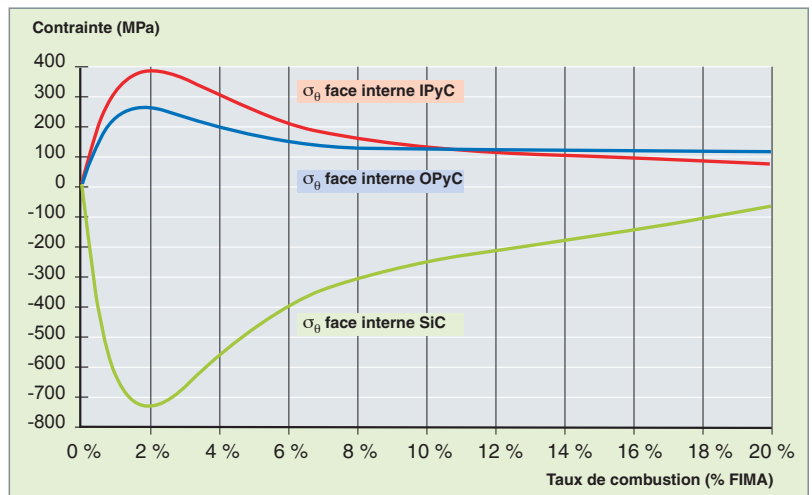
Fig. 117. Exemple de calcul d'évolution de contraintes tangentielles dans les couches IPyC, SiC et OPyC. Au début de l'irradiation, le pyrocarbone se rétracte, ce qui a pour effet de mettre la couche de SiC en compression. Plus tard, l'accumulation des PF gazeux fait monter la pression dans la particule, et le SiC passe en traction. Ce sont les contraintes de traction et non de compression qui créent les ruptures de cette couche. Sur l'exemple ci-dessus, le SiC reste en compression jusqu'à 20% FIMA, mais selon les scénarios, les particules peuvent passer en traction beaucoup plus tôt, avec des risques de rupture accrus.
