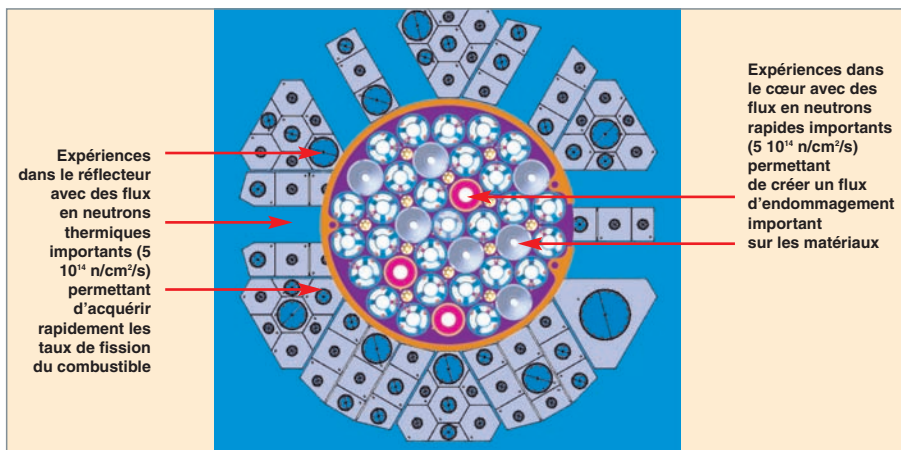
Fig. 132. le cœur du RJD est contenu dans un cylindre d'une soixantaine de cm de diamètre et de hauteur.
