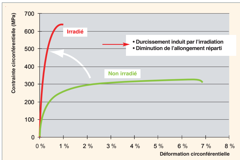
Fig. 35. Évolution du comportement mécanique en écouissage à 350 °C (essai d'éclatement) d'un alliage de Zr avant/après irradiation ( 10^{25} n/m 2 ).
