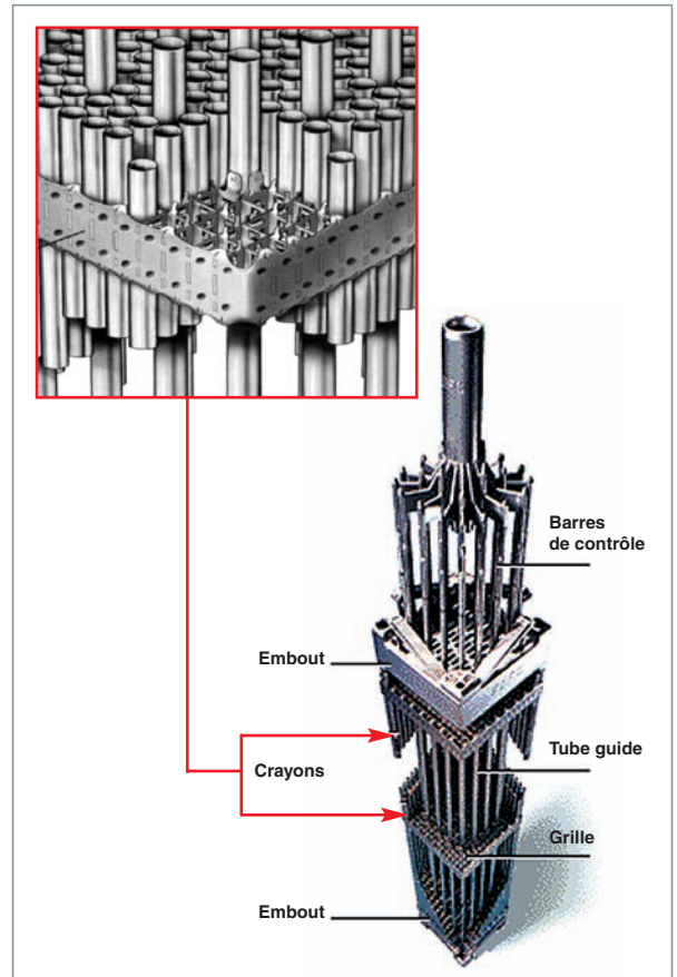
Fig. 33. Assemblage combustible des réacteurs à eau sous pression (REP).
