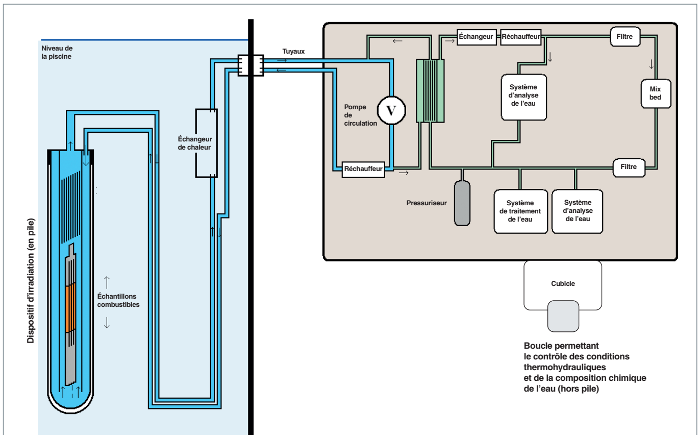
Fig. 98. Le dispositif d'irradiation MADISON, pour l'étude du comportement du combustible en conditions « normales ».
