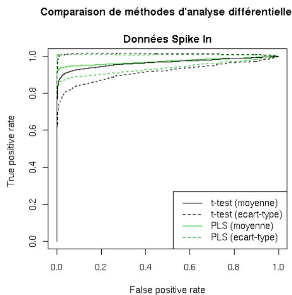
FIGURE 7 – Moyennes des différentes courbes ROC pour toutes les configurations possibles : comparaison entre le t-test et la régression PLS (sans standardisation)
